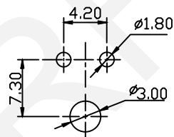
02P P.C.B Layout
