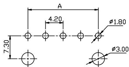
03~06P P.C.B Layout
